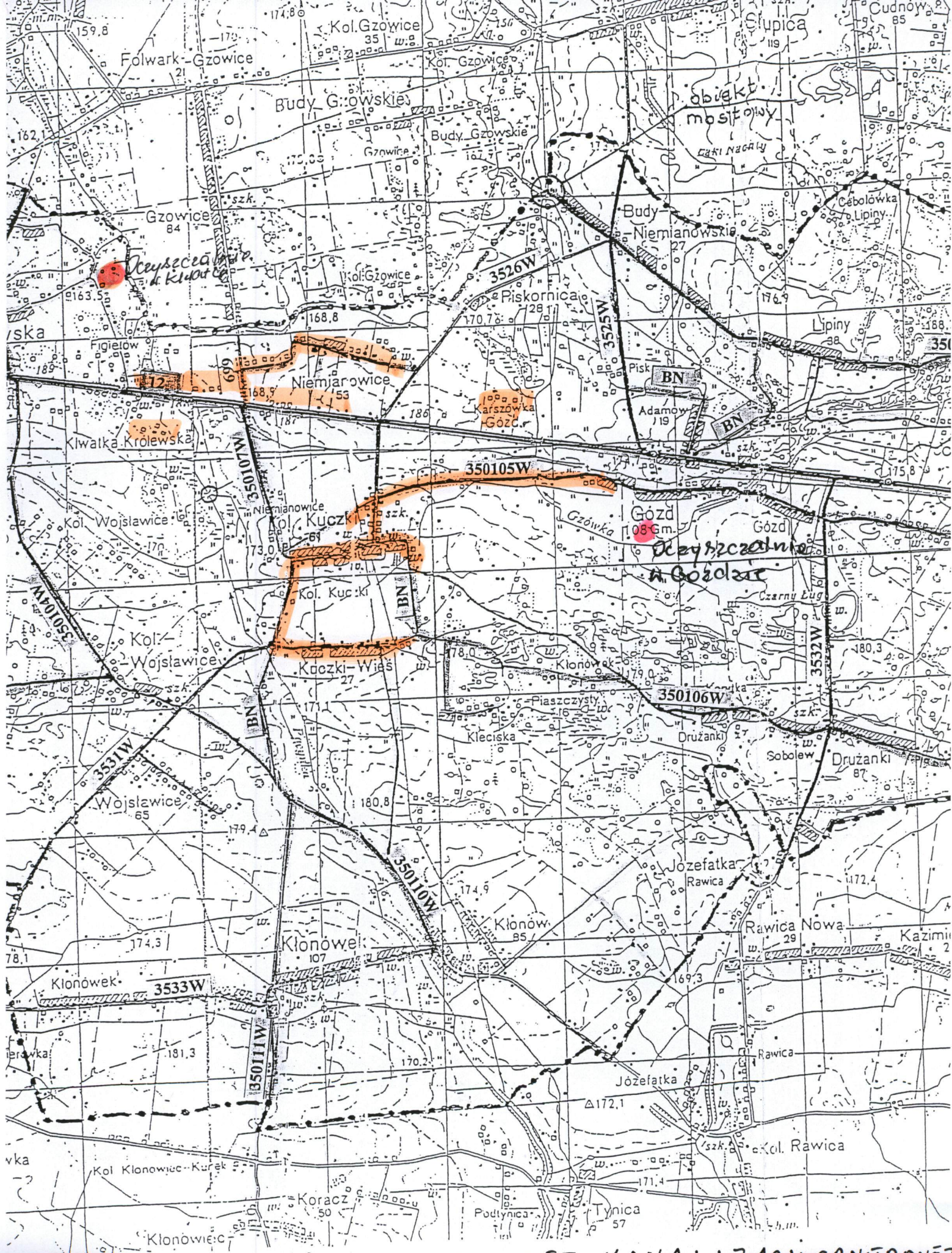
MAPA ORIENTACYJNA PROJEKTOWANEJ KANALIZACJI SANITARNEJ
