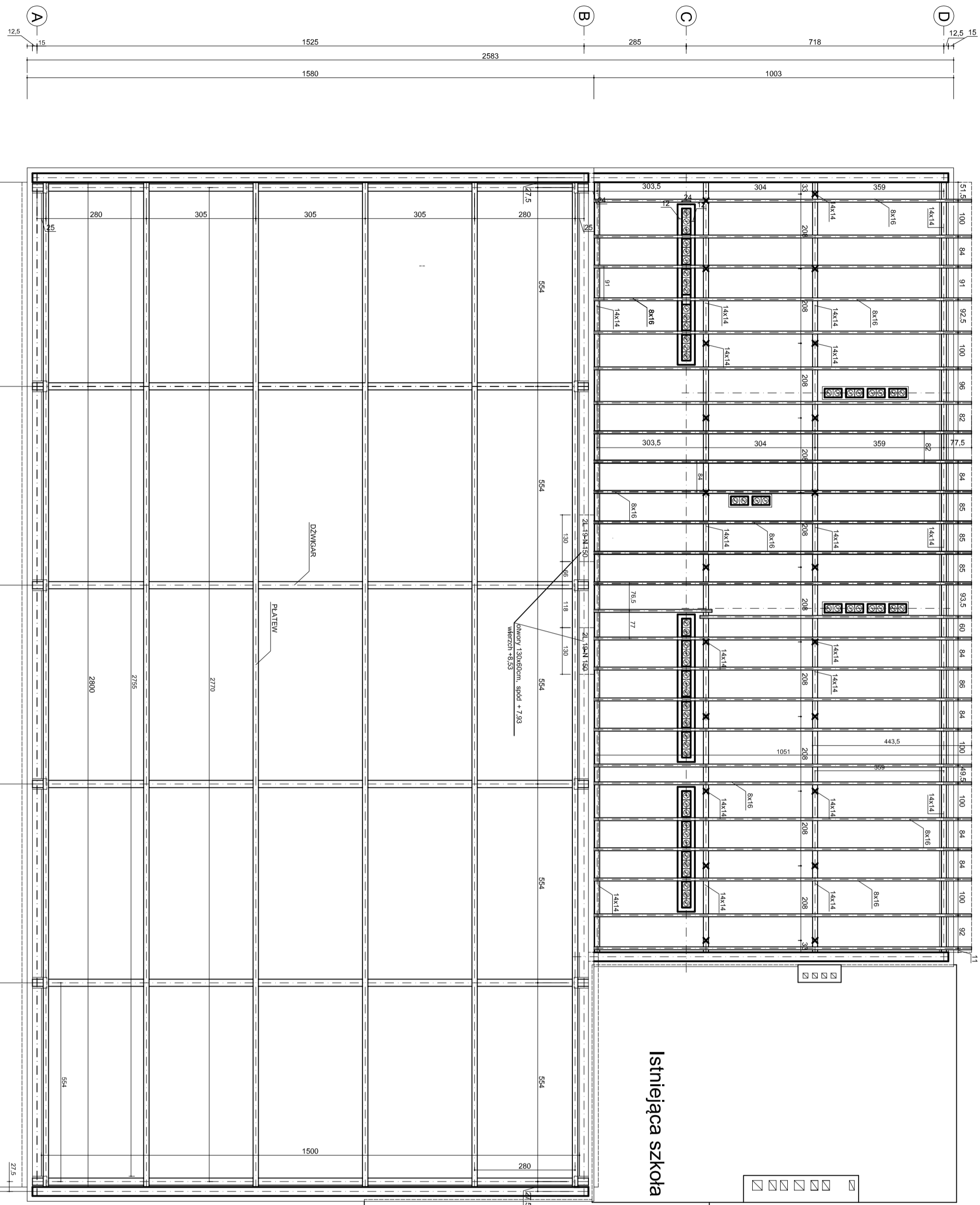
RZUT WIĘZBY I DZWIIGARÓW
